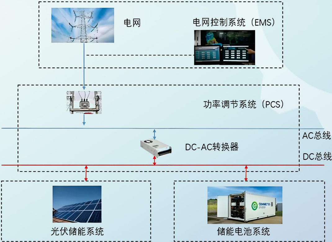
光伏储能
